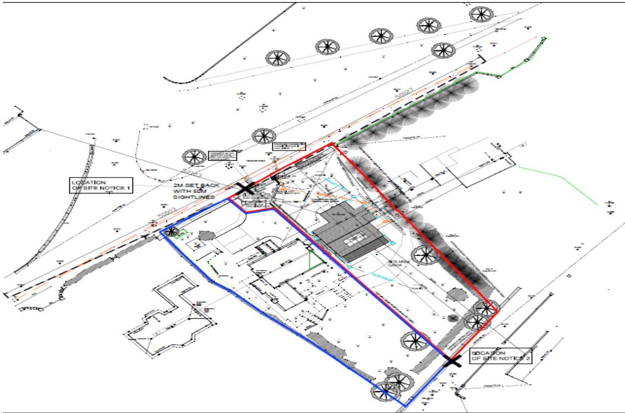
SITE PLAN 1:500
